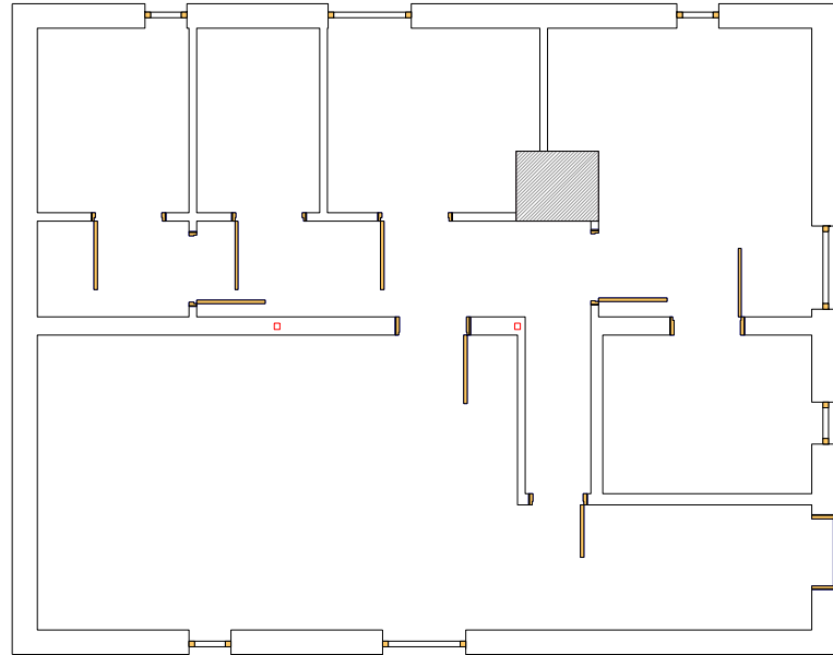
Källarplan
