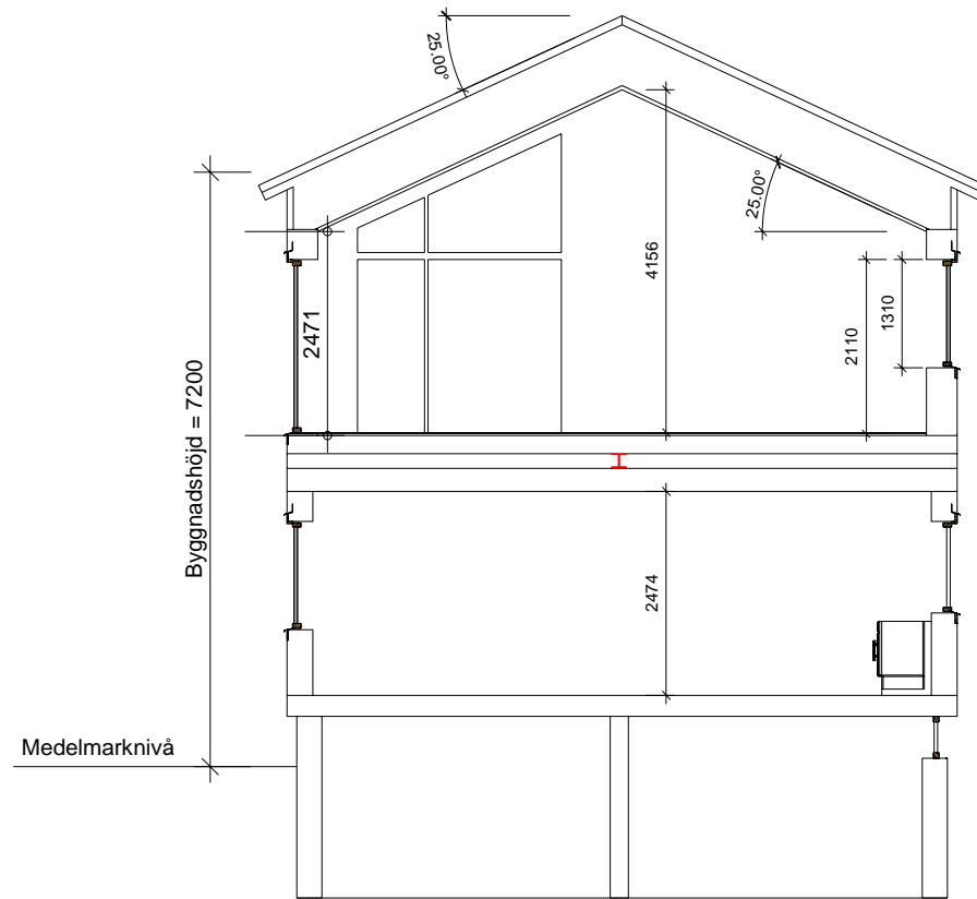
Snitt A-A
