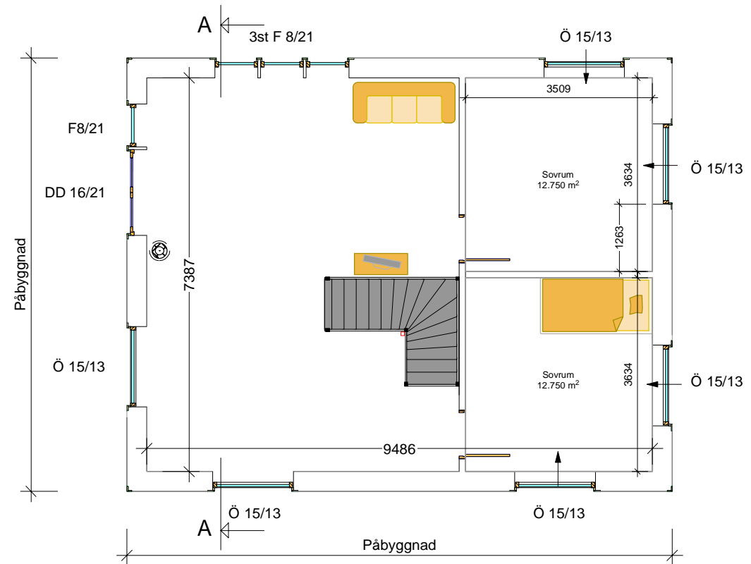
Takvåning / påbyggnad
