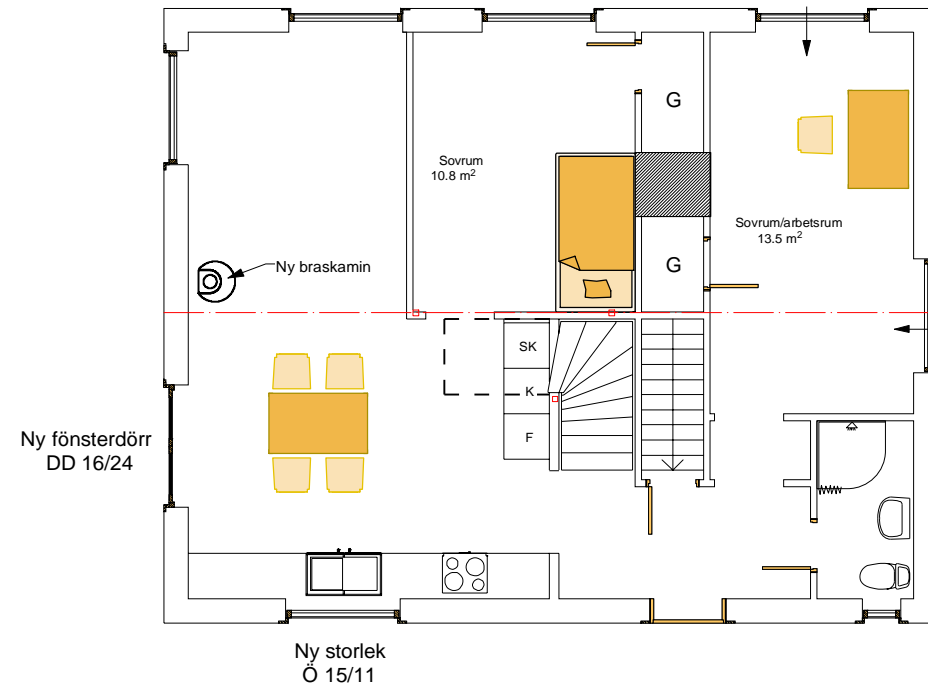
Takvåning / påbyggnad
