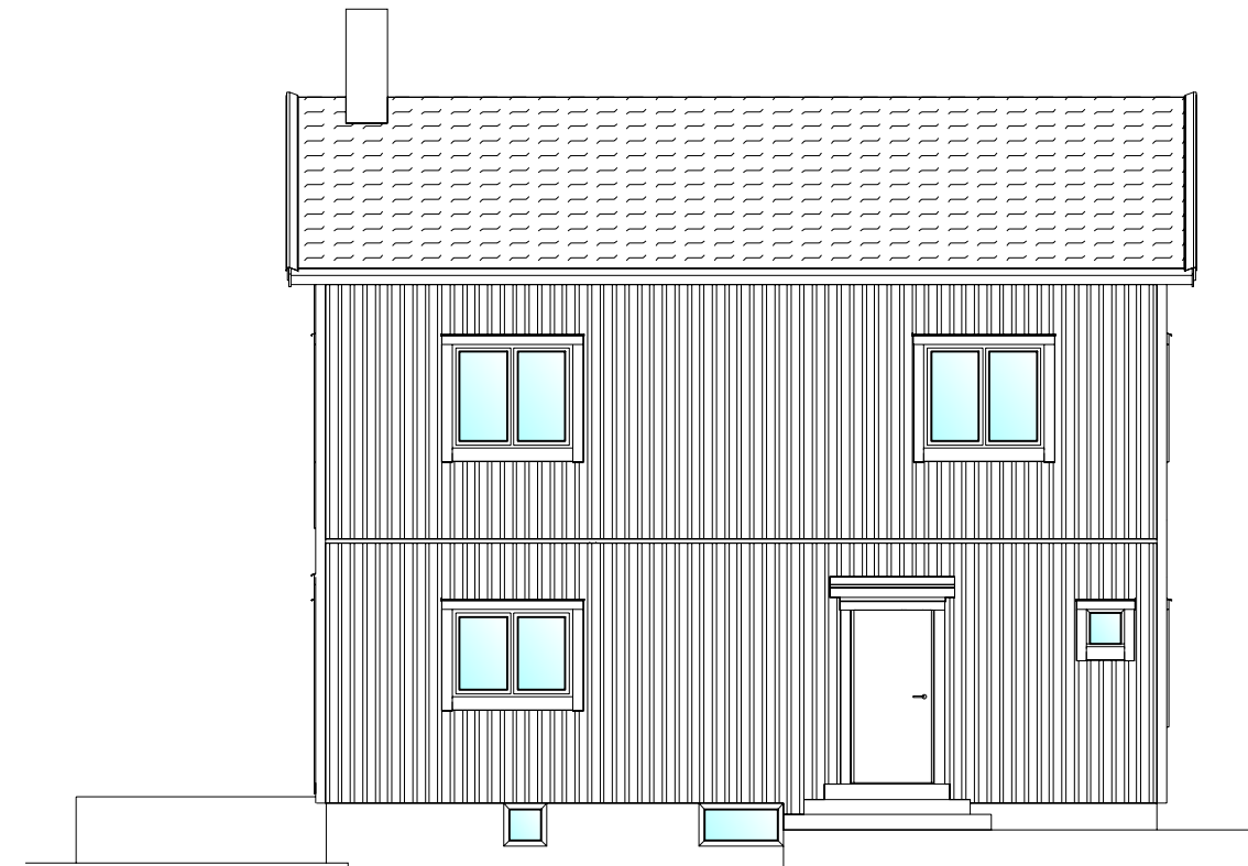
Fasad mot söder
