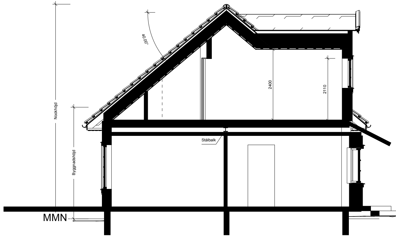
Sektion A-A
