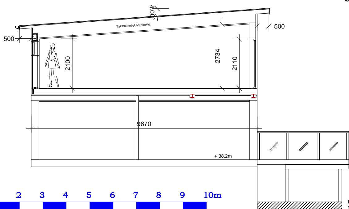
Sektion A-A
