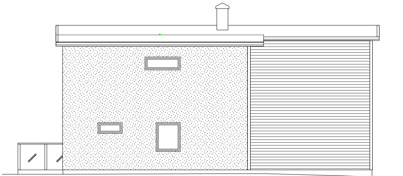
Fasad mot norr
