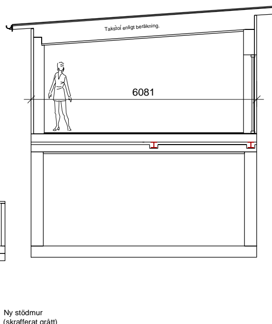
Sektion B-B
