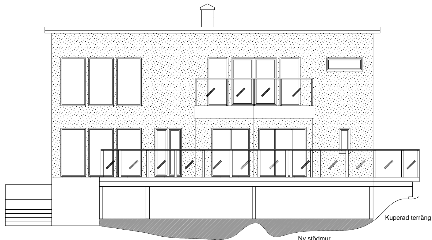
Fasad mot söder
